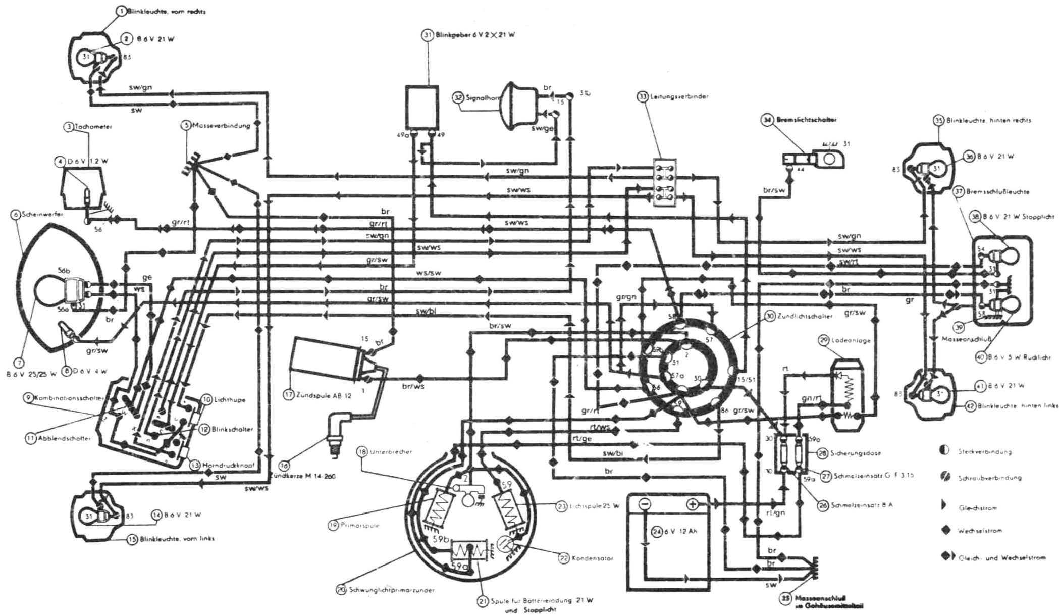
Schaltplan S51 B1-3 und B1-4
