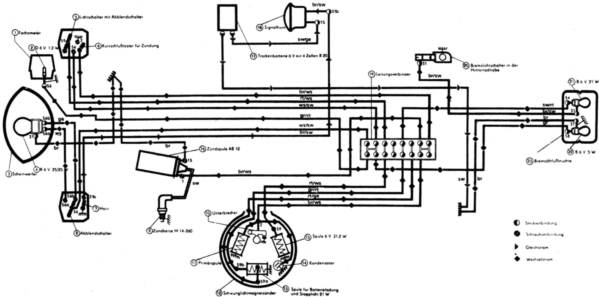
Schaltplan S51 E4
