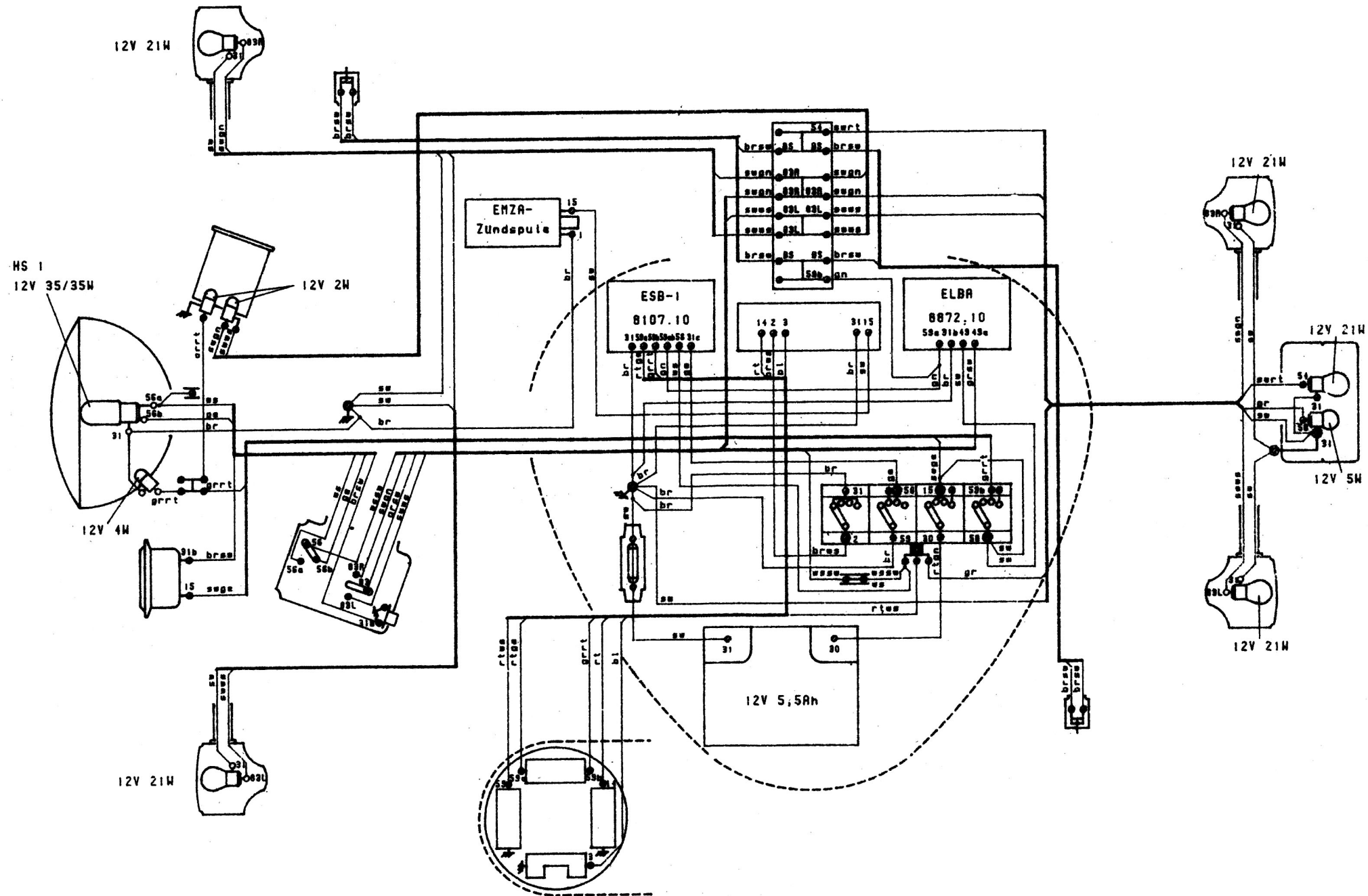
Schaltplan S51/1 C1, S51/1 E und S70/1 E
