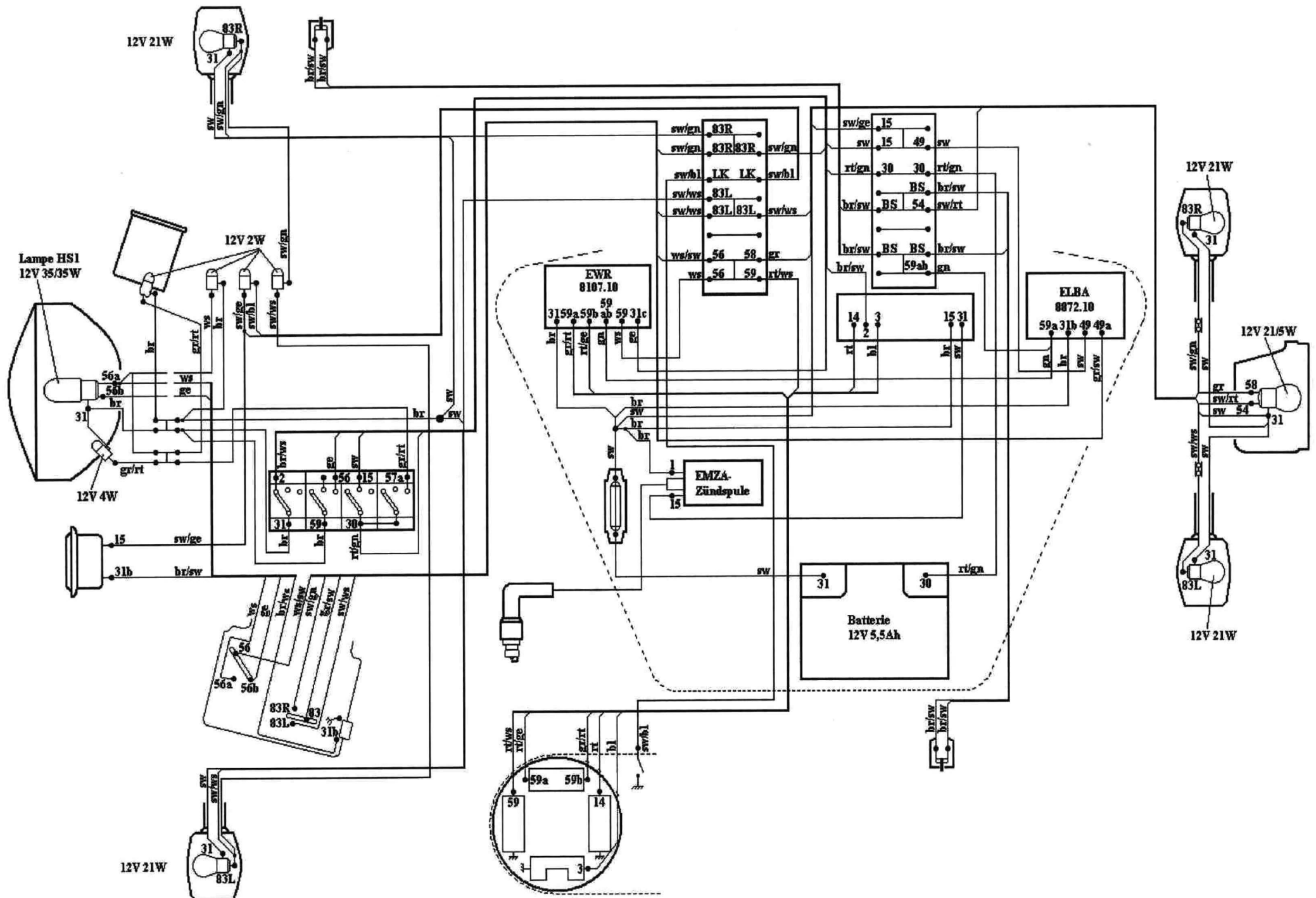
Schaltplan S 53 B und S 53 E
