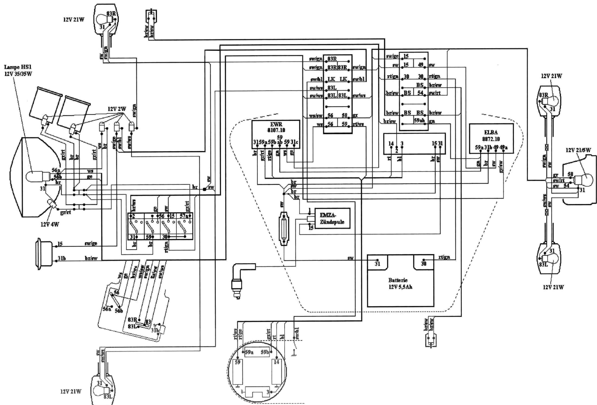
Schaltplan S 53 C
