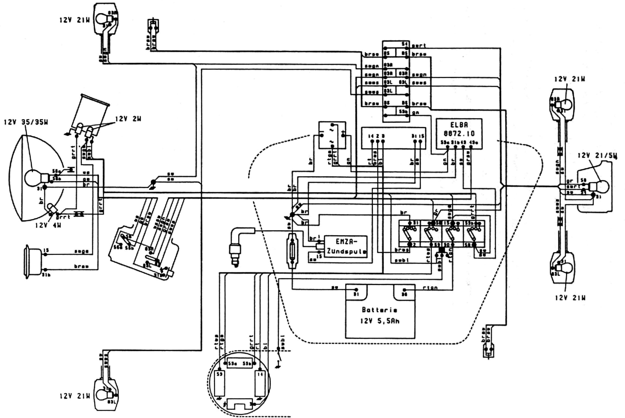
Schaltplan S53 N
