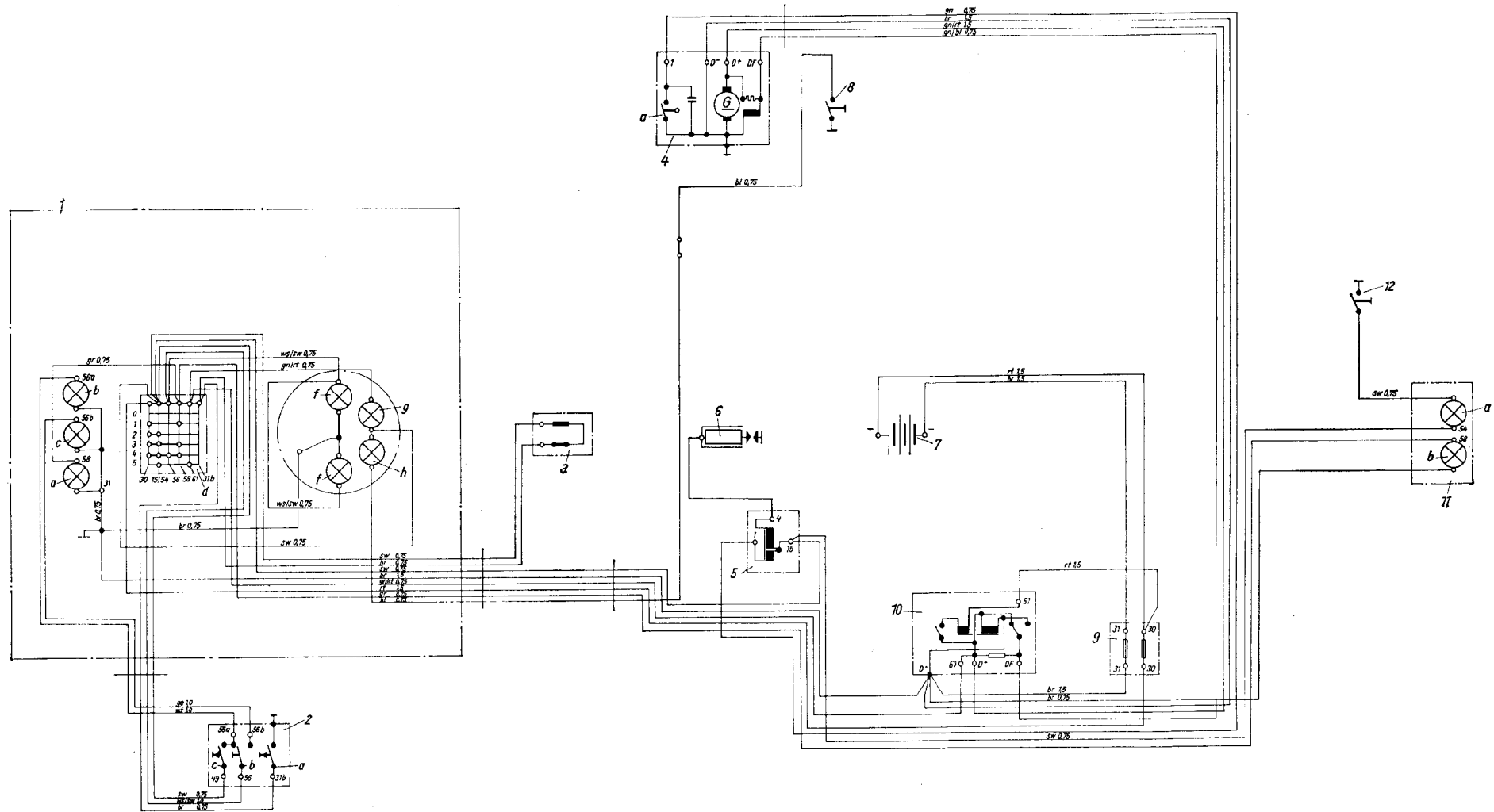
Bild 80. Schaltplan ohne Blinkleuchten (TS 125 und 150)
